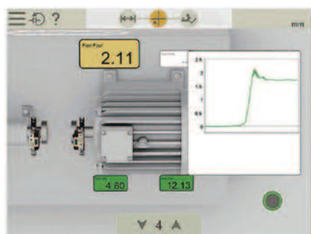
软脚检查
