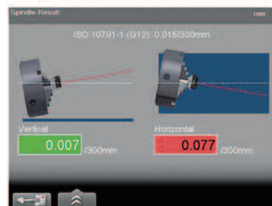
测量结果，红色超出公差
